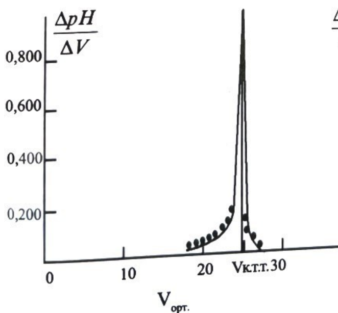
8.8.1. Күшті қышқылды күшті негізбен титрлеудің дифференциалды қисығы
