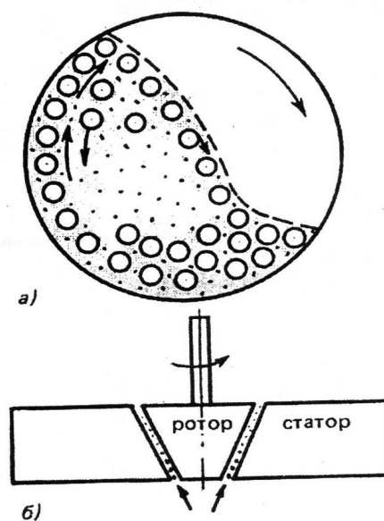
Рис. 12.2. Схемы диспергаторов: а — шаровая мельница; б — коллоид- ная мельница
