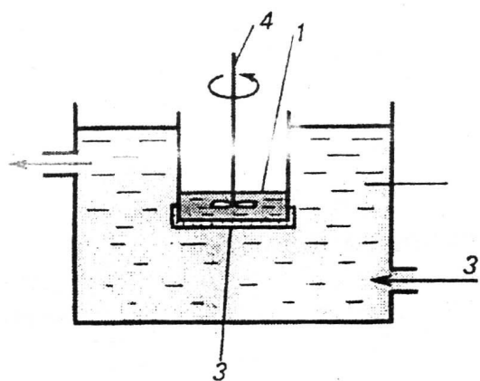
Рис. 12.3. Диализатор: 1 — диализуемая жидкость; 2 — растворитель; 3 — диализная мембрана; 4 — мешалка
