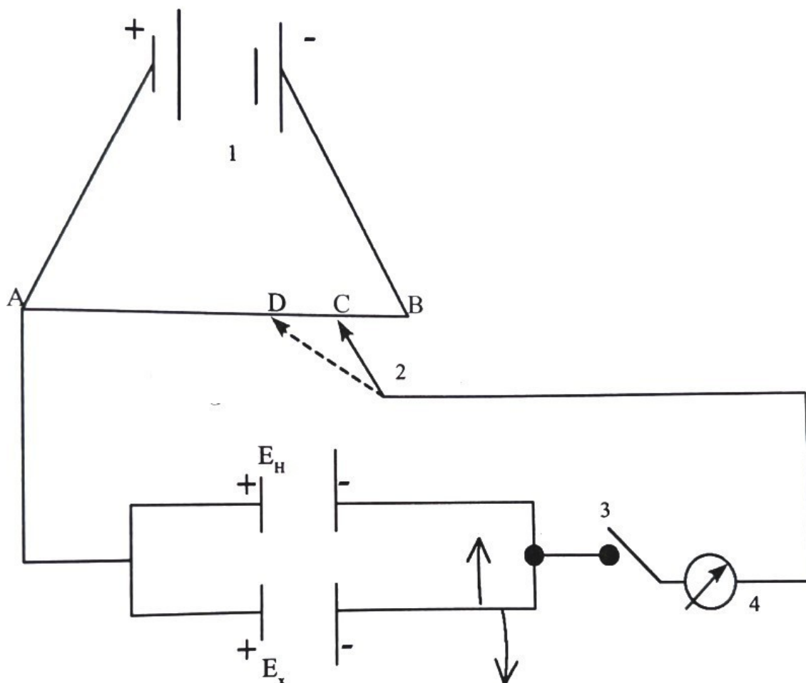
8.6. Сурет. ЭҚК өлшейтін құралдың компенсациялық сызбанұсқасы: 1- аккумулятор; 2- қозғалатын контакт; 3- кілт; 4-гальванометр
