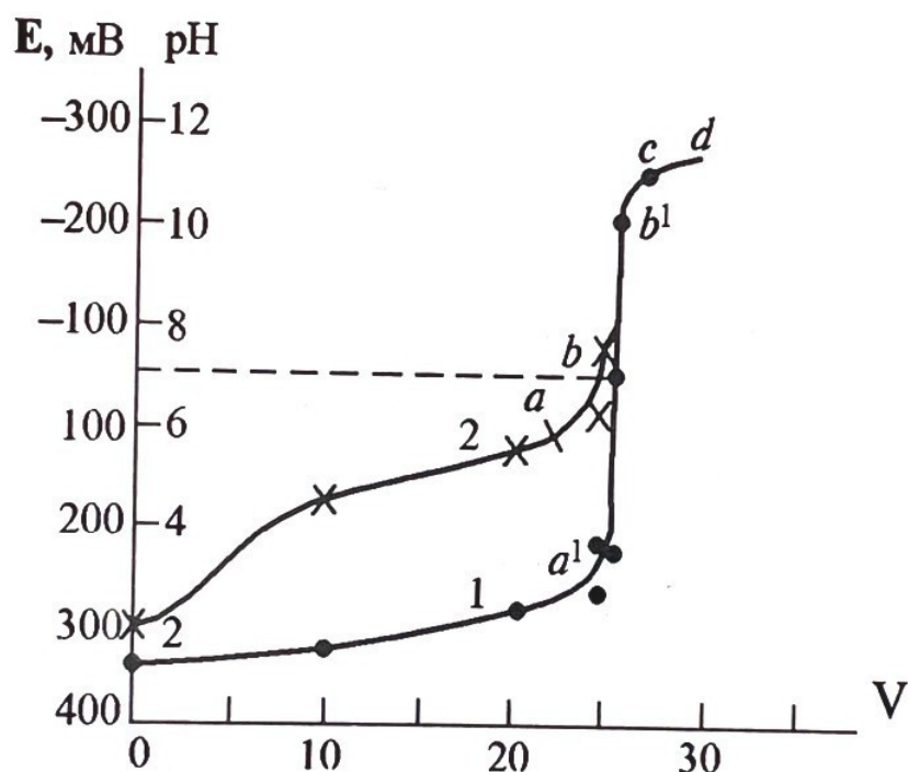
8.9. сурет. Потенциометрлі титрлеуді интегралды қисығы 1- күшті қышқыл, 2-әлсіз қышқыл
