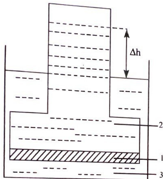
5.1.5. сурет. Осмометр: 1 – жартылай өткізгіш мембрана 2 – ерітінді бар ыдыс 3 – еріткіш су бар ыдыс.
