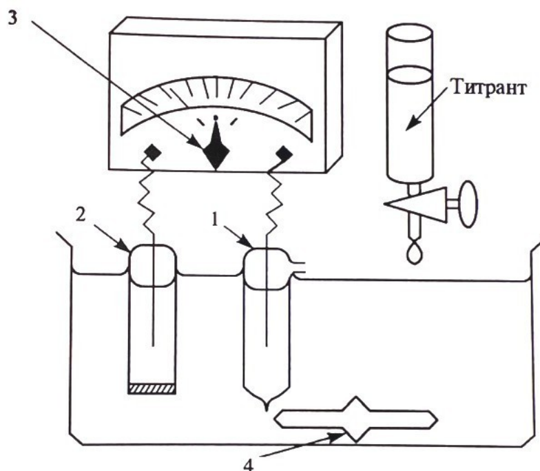
8.7. сурет. Потенциометрлі титрлеу. 1 – салыстырушы электроды (хлоркүмісті); 2 - анықтаушы электрод (шыны); 3 - диапазондарды ауыстырғыш; 4- магниттік араластырғыш.
