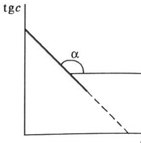
10.2. 2. сурет. Бірінші ретті реакция үшін концентрация логарифмнің уақытқа тәуелділігі
