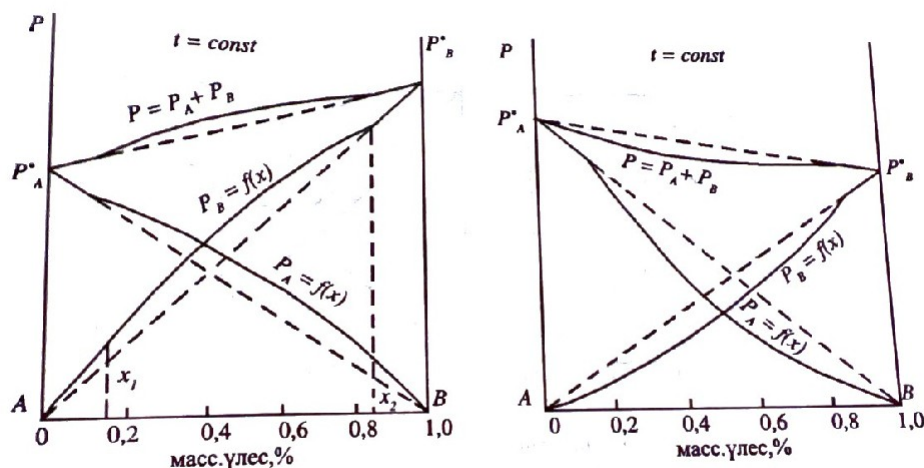
6.3.1. сурет. Қаныққан бу қысымның жүйе құрамына тәуелділігінің Рауль заңынан ауытқуы; а-оң, б-теріс.
