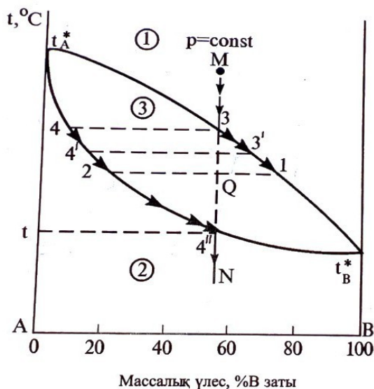
4.5.3. Қатты және сұйық кезінде өзара шексіз еритін жүйелер.
