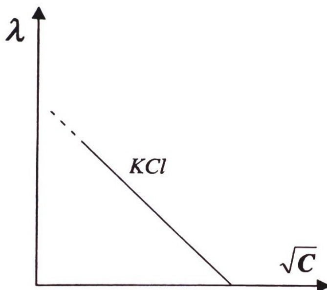
7.5. Сурет. Молярлы электроөткізгіштіктің концентрацияға тәуелділігі ( \lambda - \sqrt{C} )
