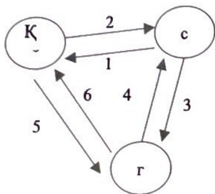
4.3. сурет. Фазалар ауысу схемасы
