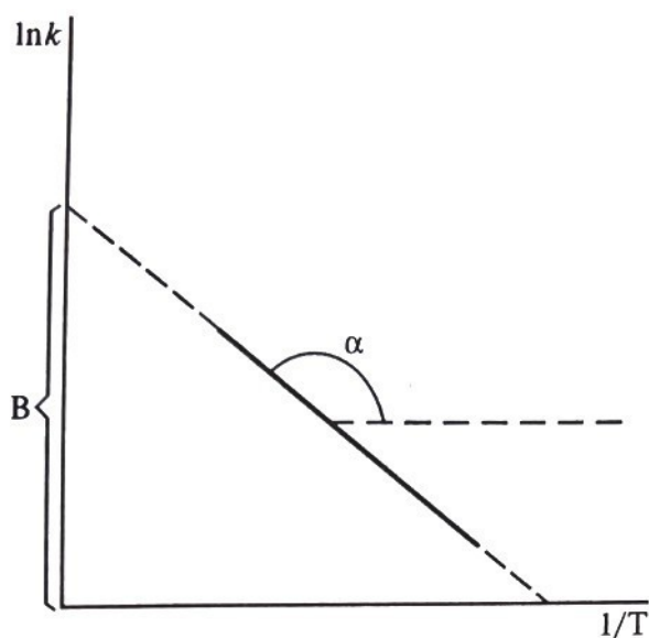
10.4. сурет. Аррениус коэффициентерін тәжірибелік анықтау әдістері
