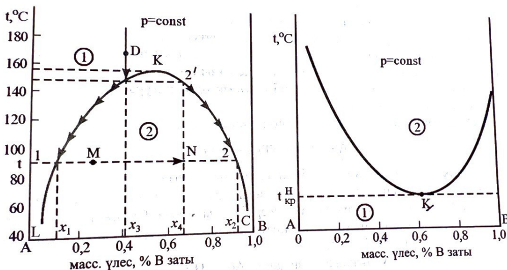
6.5. сурет. Ерудің дағдарыстық температуралары бар өзара шекті еритін сұйықтардың күй диаграммасы: а-жоғары; б-төменгі
