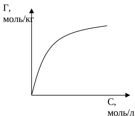
1.2.2. Сурет. Фрейндлих теориясының адсорбция изотермасы
