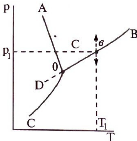
4.4. сурет. Бір компонентті жүйелердің (су, күкірт) күй диаграммалары. Фазалар ережесін қолдану
