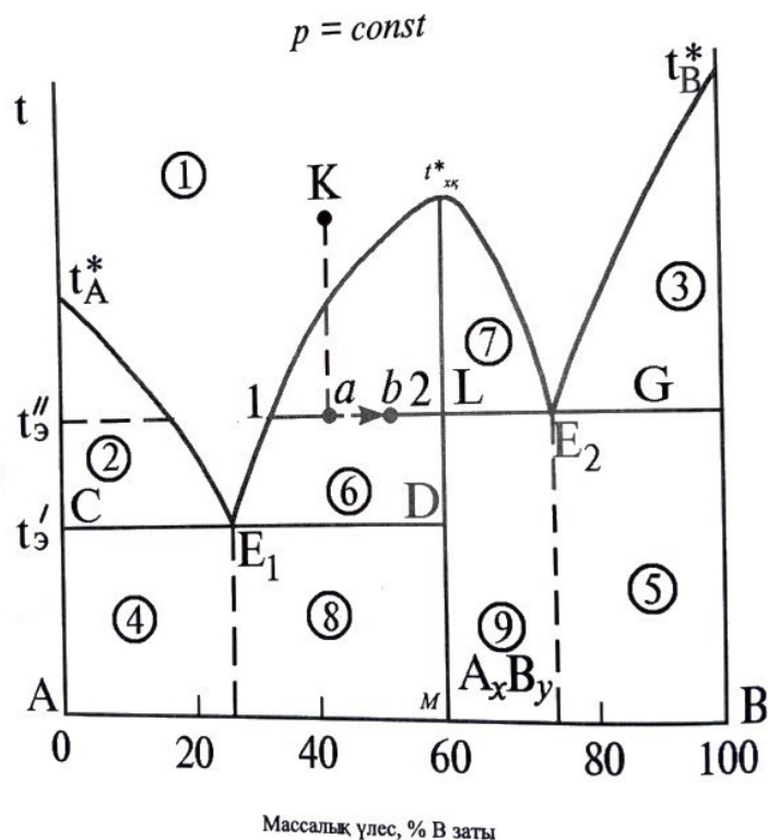
4.5.2. сурет. Конгруэнтты балкытын химиялық қосылысы бар екі компонентті жүйенің диаграмасы.
