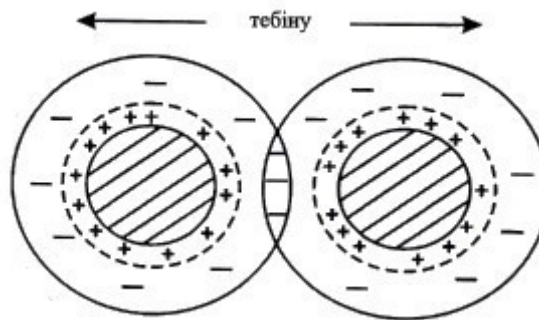
13.2.9. сурет. Коллоидты ерітінділердің тұрақты болу механизмі.
