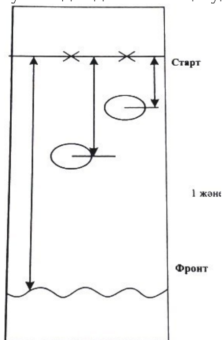
12.3.2. Хроматограмма. 1 және 2 компоненттердің орналасуы.
