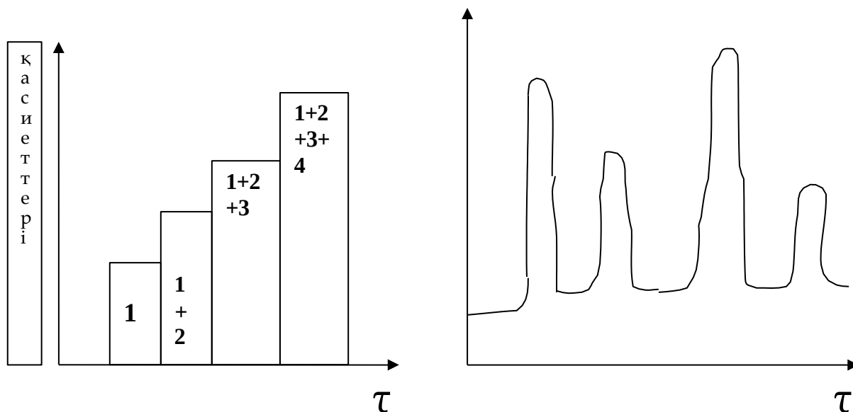
12.3.1. Хроматографиялық зоналарға сорбция изотермаларының әсері
