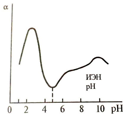
15.7. Сурет. Ісіну дәрежесінің рН-қа тәуелділігі
