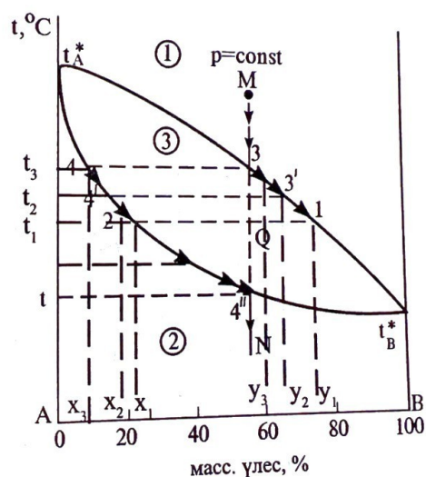
6.4.3. сурет. Бу және сұйық фазаларының құрам тепе-теңдігінің жай айдаудан кейін өзгеруі
