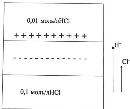
8.1. сурет. Диффузиялық потенциалдың пайда болуы
