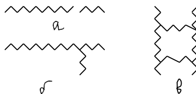
15.1. Сурет. Полимер макромолекулалар құрылысының сызбанұсқасы: а- сызықты; б- тармақталған; в- кеңістік
