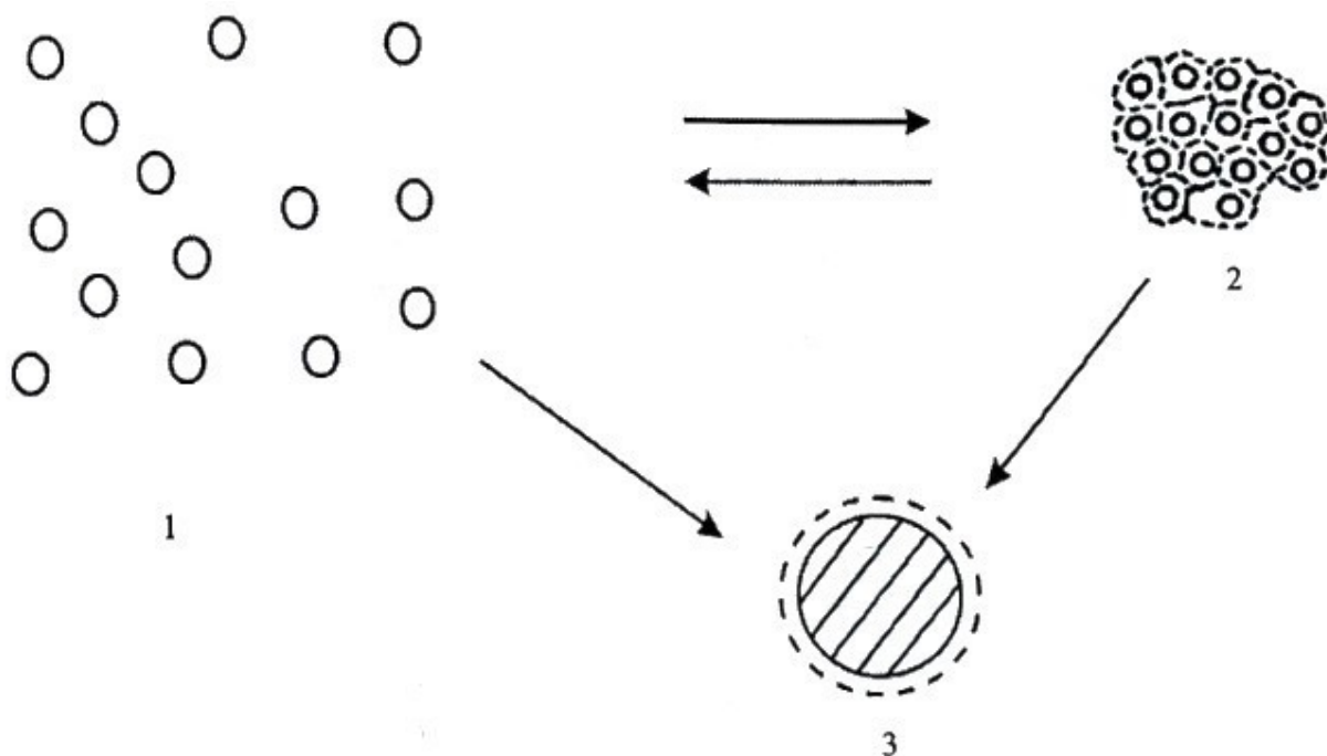
13.2.8. сурет. Дисперсті жүйелердің тұрақтылық түрлері:
