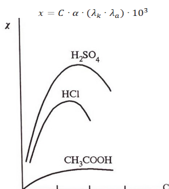
7.2. Сурет. Кейбір электролит ерітінділерінің электр өткізгіштіктерінің концентрацияға тәуелділігі
