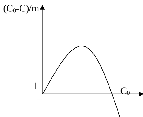
1.2.4. Ерітіндіден жүретін адсорбциясының изотермасы.
