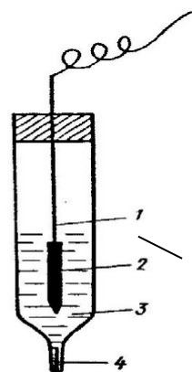
Хлорсеребряный электрод: 1 — серебряная проволока; 2 — слой AgCl; 3 — пористый материал; 4 — отверстие.
