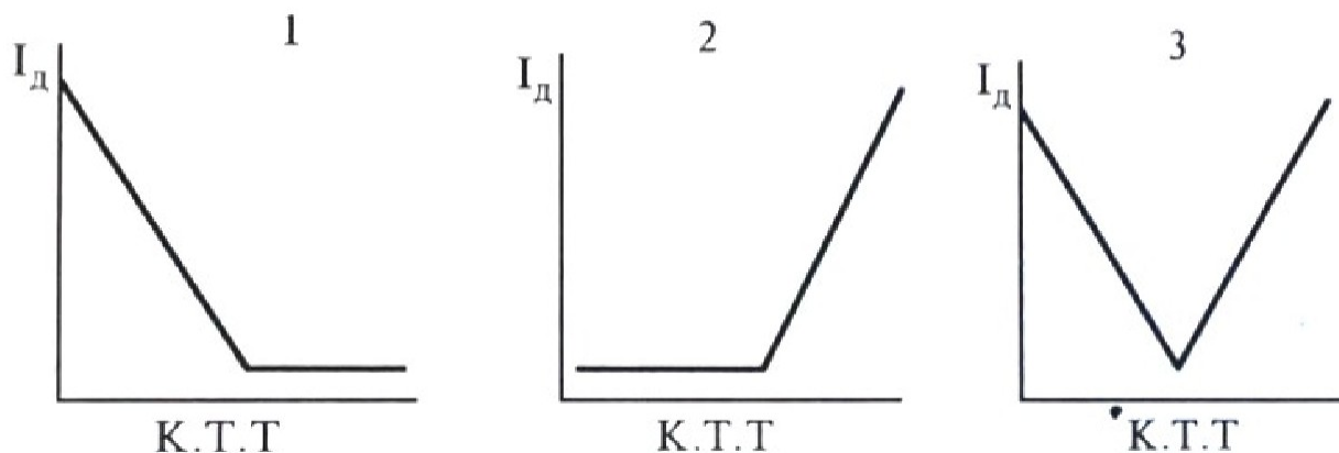
9.3. Сурет. Амперометриялық титрлеудің қисықтары
