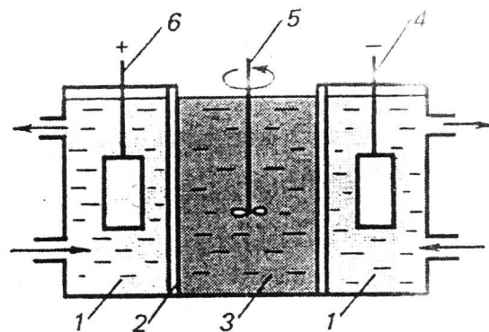
Рис. 12.4. Электродиализатор: 1 — растворитель; 2 — диализная мембрана; 3 — диализуемая жидкость; 4 — катод; 5 — мешалка; 6 — анод
