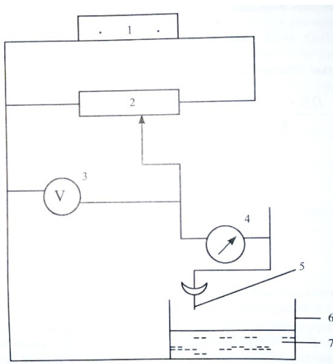
9.1. Сурет.Қарапайым полярографиялық құралдың сызбанұсқасы. 1- кернеу көзі; 2- ауыспалы кедергі; 3-вольтметр; 4-микроамперметр (гальванометр); 5- сынап тамшылайтын электрод (СТЭ); 6- полярографиялық ұяшық; 7- қосымша электрод.
