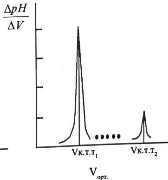
8.8.2. Күшті және әлсіз қышқылдар қоспасының титрлеуінің дифференциалды қисығы
