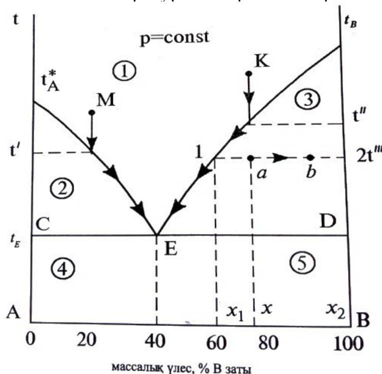
4.5. сурет. ( p = \text{const} ) А және В компоненттерінің өзара қатты күйінде ерімейтін балқу диаграммасы.
