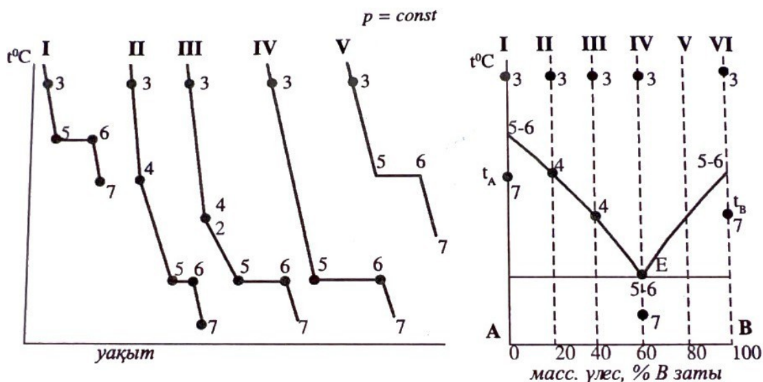
4.6. Күй диаграммаларын тұрғызу принциптері: а) салқындау қисықтары; б) – күй диаграммасы
