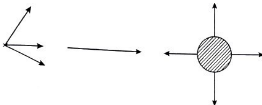
13.2.3. Сурет. Ультрамикроскоптан шар тәрізді бөлшектің көрінуі.
