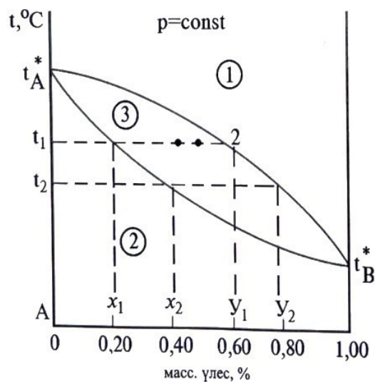
6.2.2. сурет Идеалды бикомпонентті жүйенің қайнау диаграммасы
