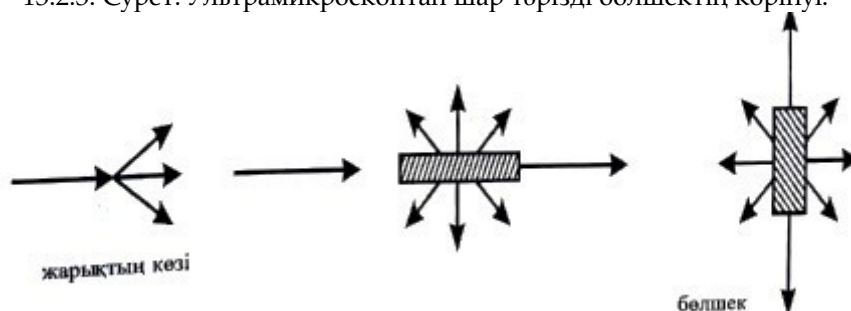
13.2.4. Сурет. Ультрамикроскоптан пластинка, таяқша, эллипсоид тәрізді бөлшектердің көрінуі.
