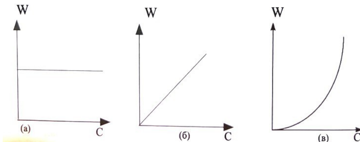
10.3. Сурет. Бірінші (а) және екінші (б) ретті реакция үшін концентрацияның уақыт бойынша өзгеруі
