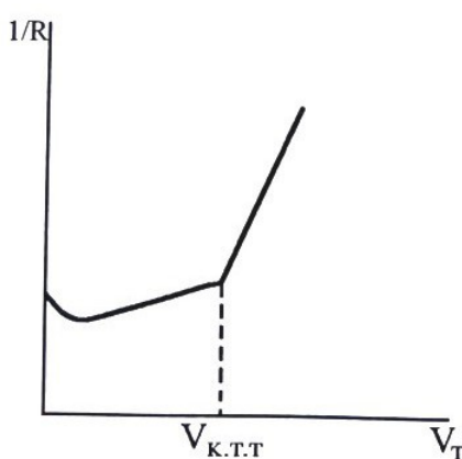
7.7.2. сурет. Әлсіз қышқылды күшті негізбен титрлеудің кондуктограммасы
