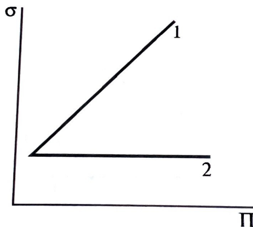
1.1.2. Сұйықтық-газ жүйесіндегі беттік керілудің сұйық фазасының полярлығына тәуелділігі
