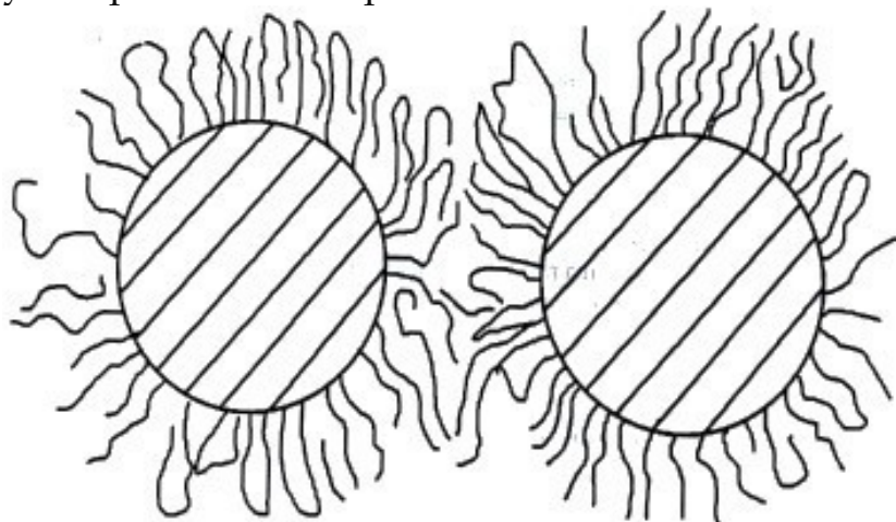
13.3.3-сурет. Коллоидты қорғаудың механизмі
