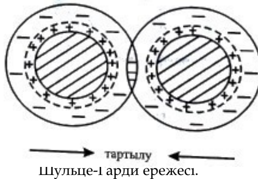
13.2.9. сурет. Коллоидты ерітінділердің тұрақты болу механизмі.
