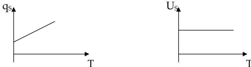
1.1.3. Сурет. Беттік энергияның температураға тәуелділігі: а) аудан бірлігінің түзілу жылуы; б – толық энергия
