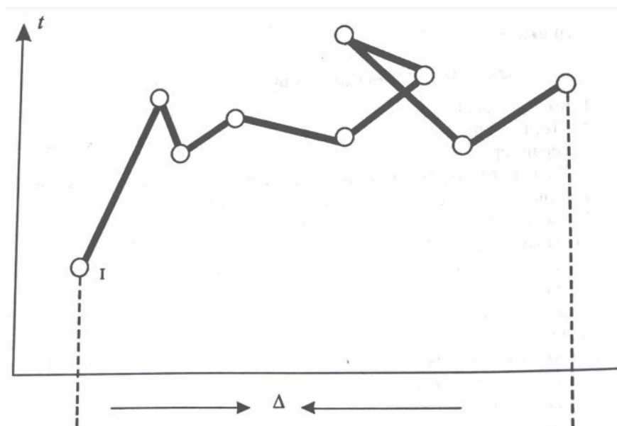
13.2.1-сурет. Броун қозғалысында бөлшектің орын ауыстыру сызбанұсқасы. \Delta x – 1 нүктеден 2-нүктеге дейін орын ауыстыруының шамасы, t – уақыт.
