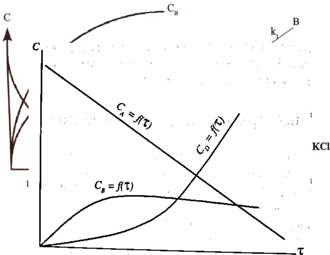
10.5. Кезектес реакциялар үшін әрекеттесуші заттар концентрацияларының уақыт бойынша өзгеруі.
