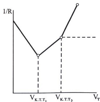
7.7.3. сурет. Күшті және әлсіз қышқылдар қоспасын күшті негізбен титрлеу кондуктограммасы
