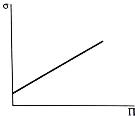
1.1.4. Сурет. Сұйықтық-сұйықтық жүйесінде беттік керілудің фазалар полярлығының айырмашылығына тәуелділігі
