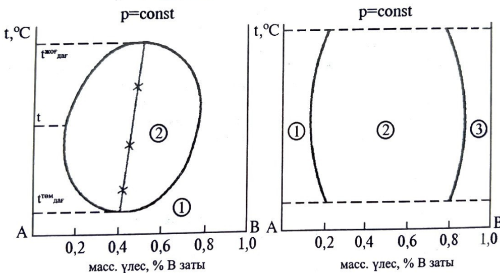
6.6. сурет. Өзара шекті еритін сұйықтардың күй диаграммасы: а-жоғары және төменгі ерудің дағдарысты температураларымен; б-ерудің дағдарыстық температураларынсыз
