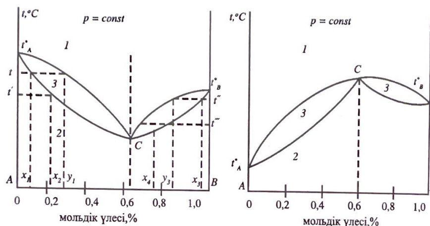
6.4.2. сурет. Ерітінді қайнау температурасының құрамға тәуелділігі: а – бу қысымының қисығында минимумы бар жүйелерге; б – бу қысымының қисығында максимумы бар жүйелерге
