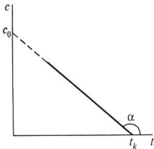
10.2. 1. сурет. Нөлінші ретті реакция үшін концентрацияның уақыт бойынша өзгеруі
