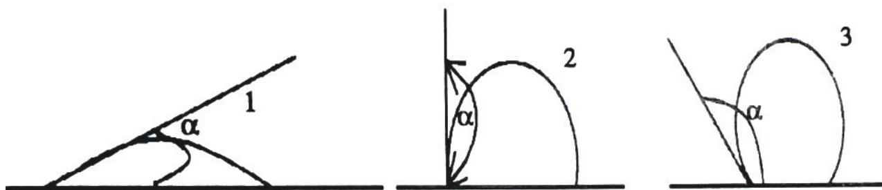
12.2.7. Шекті жұғу бұрышы:
