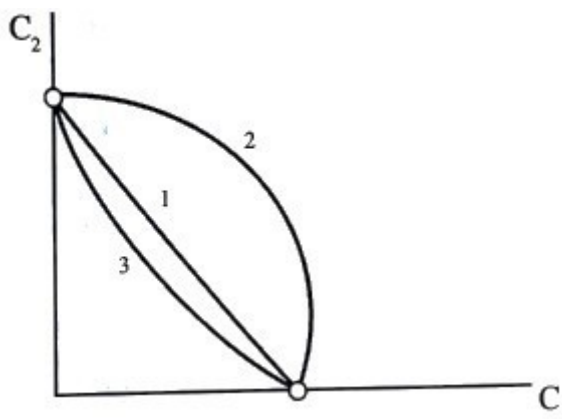
13.3.2-сурет. Электролиттер қоспасымен коагуляциялау әсері:
