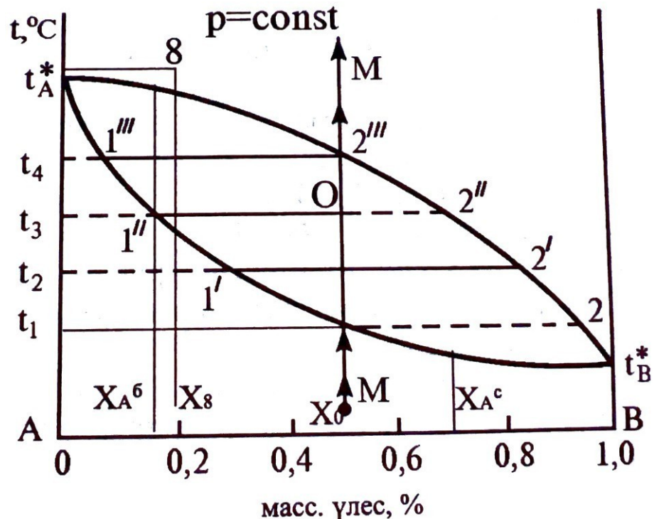
6.2.3. сурет. Идеалды екі компонентті жүйенің қайнау диаграммасының анализі (температура-құрам).
