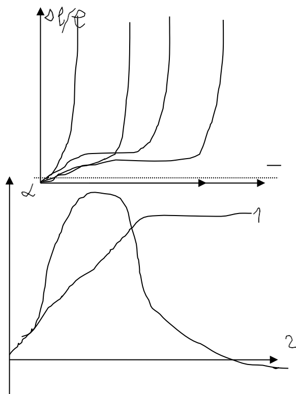
15.4. Ісінуінің кинетикалық қисықтары: 1- шекті ісіну; 2- шексіз ісіну x - өсі бойынша уақыт, y - ісіні дәрежесі ( \alpha )
