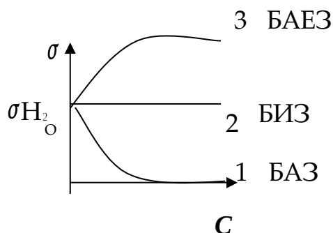
1.1.5. Сурет. Судың беттік керілу шамасына еріген заттың әсері. 1- БАЗ; 2-БИЗ; 3-БАЕЗ.
