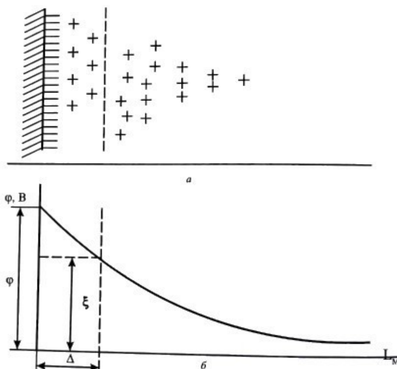
13.9. Қос электр қабаты: а - зарядтардың таралуы; б - электрокинетикалық потенциалдың кемуі.
