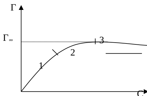
12.2.1. Сурет. Лэнгмюр теориясының адсорбция изотермасы.
