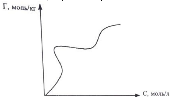
12.2.3. Сурет. БЭТ теориясының адсорбция изотермасы.
