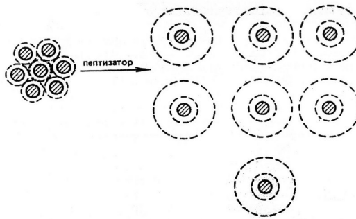
Рис. 12.18. Механизм пептизации
