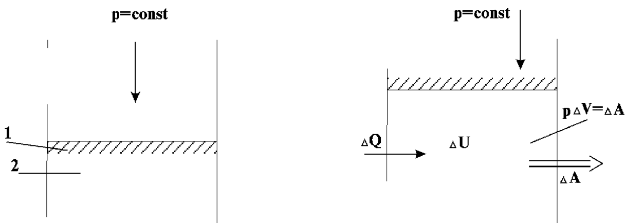
1.1. сурет. Термодинамиканың бірінші бастамасының математикалық өрнектелуін түсіндіретін сызба-нұсқасы.
