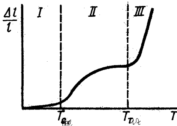
15.2. Сурет. Термомеханикалық қисық
