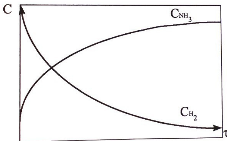
10.1. Сурет. Келтірілген реакцияның әрекеттесуші заты ( H_2 ) және өнімі ( NH_3 ) бойынша кинетикалық қисығы
