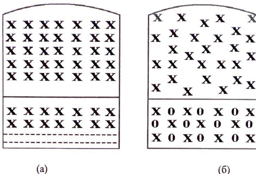
5.1.4.1. Сурет. Таза еріткіштен (а) және ерітіндіден (б) еріткіштің булануы x - еріткіш молекулалары (су), o - еріген зат молекулалары.
